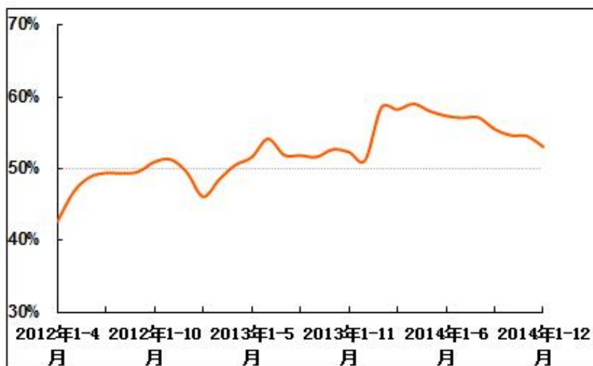
2012年-2014年电网基本建设投资占电力基本建设投资完成额比重走势
