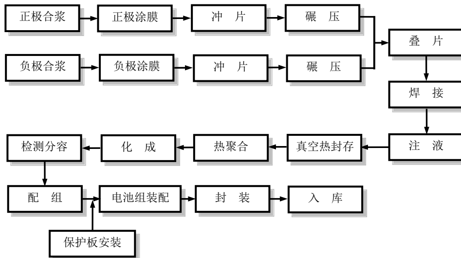
(2) 聚合物锂离子电池生产工艺流程图
