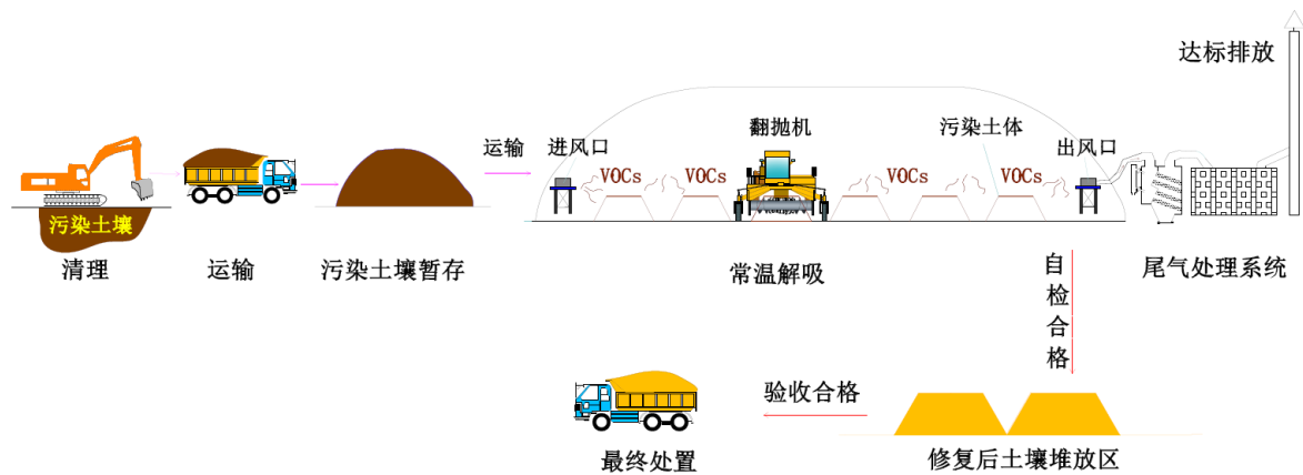
常温解吸技术工艺流程示意图
