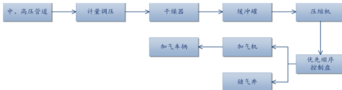
(2) CNG 标准站销售流程图
