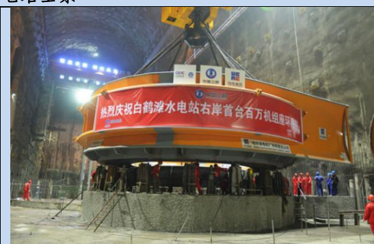
白鹤滩右岸首台机组座环吊装
