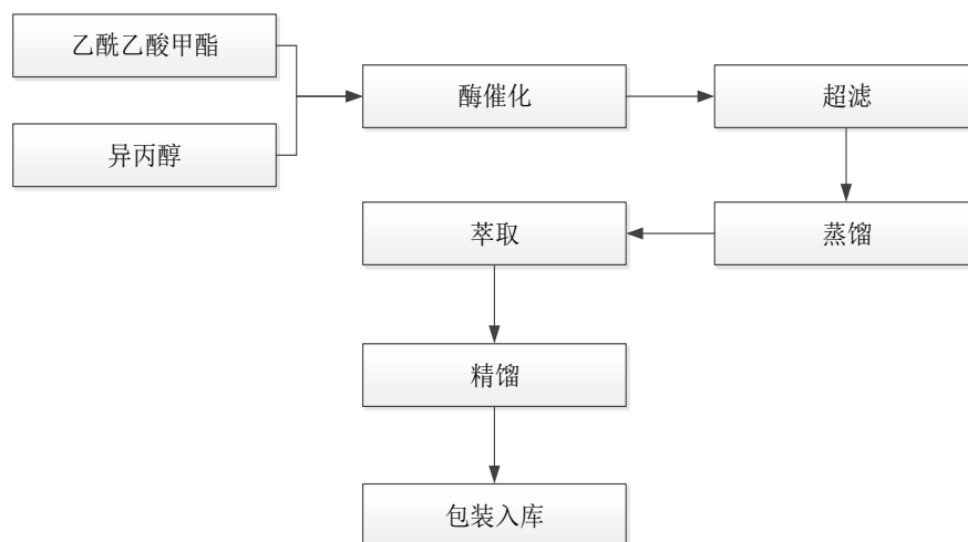
7) R-3-羟基-4-氧基丁酸乙酯工艺流程图
