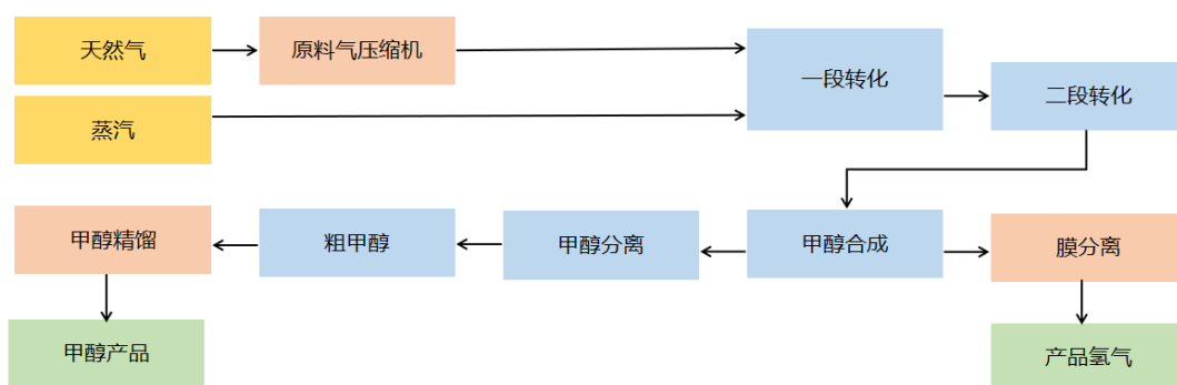
甲醇的生产工艺流程图
