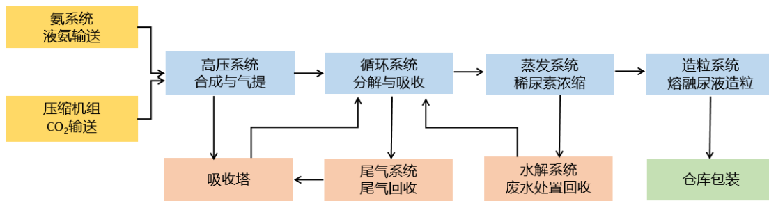
复合肥的生产工艺流程图
