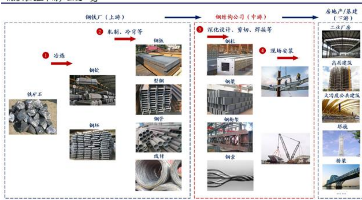
钢结构及上下游产业链一览
