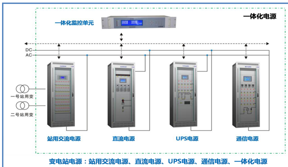
附：站用电源系统图
