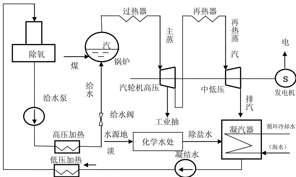
(4) 发电业务流程图
