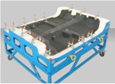
⑤内前围检具
