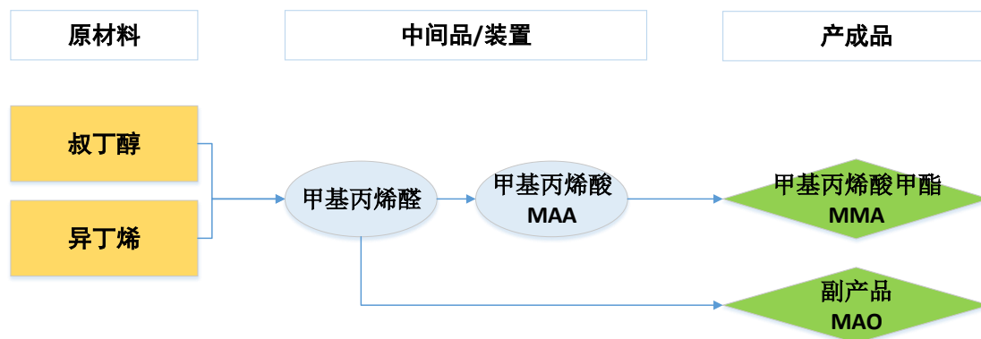
图：菏泽华立生产流程图
