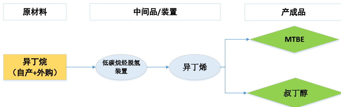
图：齐翔腾达局部生产流程图
