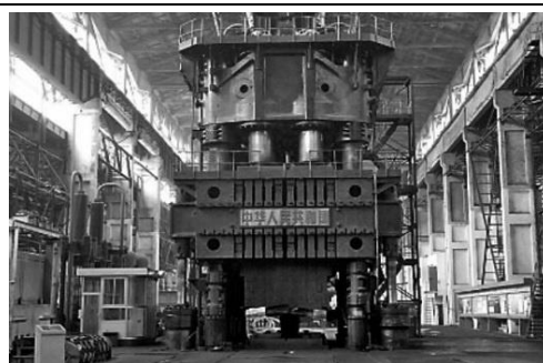
西南铝业 300MN 液压机
