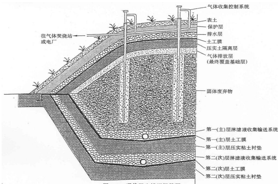
图 1.1 现代卫生填埋场库区简图
