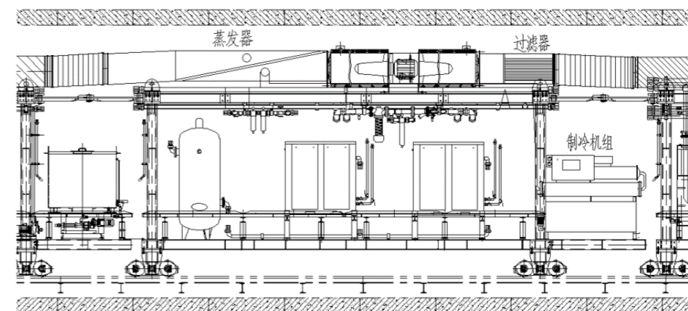
盾构机智能冷风系统。
