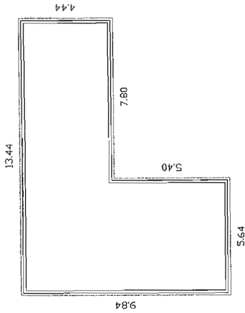
第5幢第1层平面图
