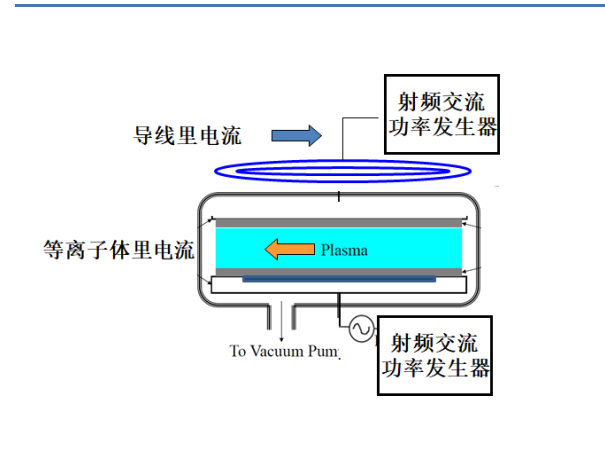
电感性等离子体刻蚀反应腔
