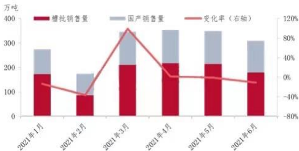
图 2 2021 年上半年 LNG 消费量走势图（数据来源于：隆众资讯）
