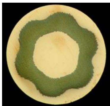
NbTi 超导线
