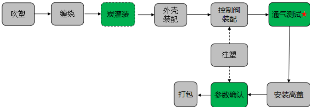
(3) 净水机生产工艺流程图
