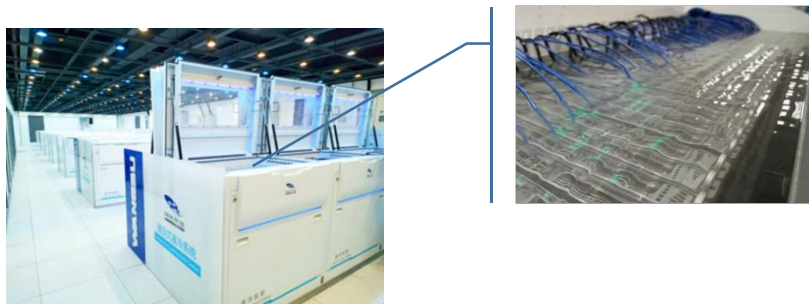
绿色云图液冷机柜
