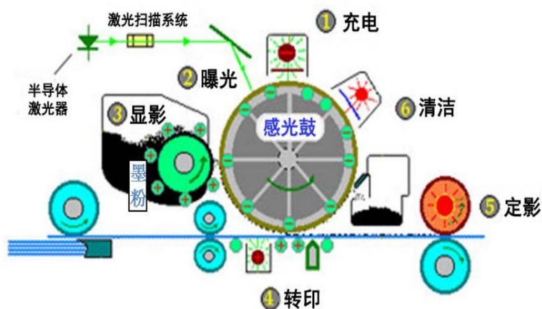
图：有机光导鼓静电成像过程
