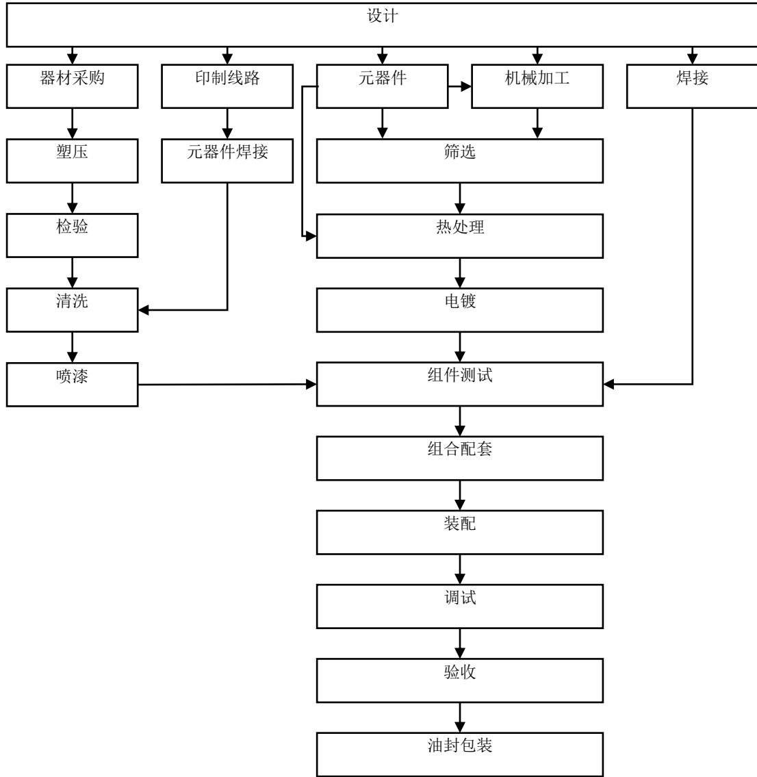
(1) 航空机载燃油测量控制系统工艺流程图
