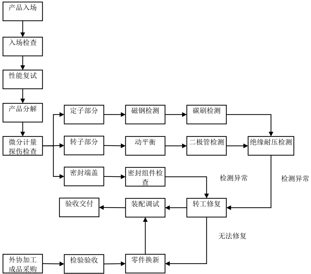
(2) 机械液压类产品维修服务工艺流程图
