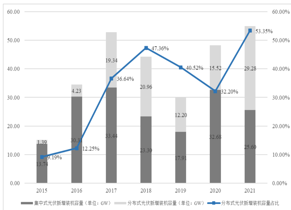
2015年-2021年我国光伏发电新增装机容量（资料来源：国家能源局）
