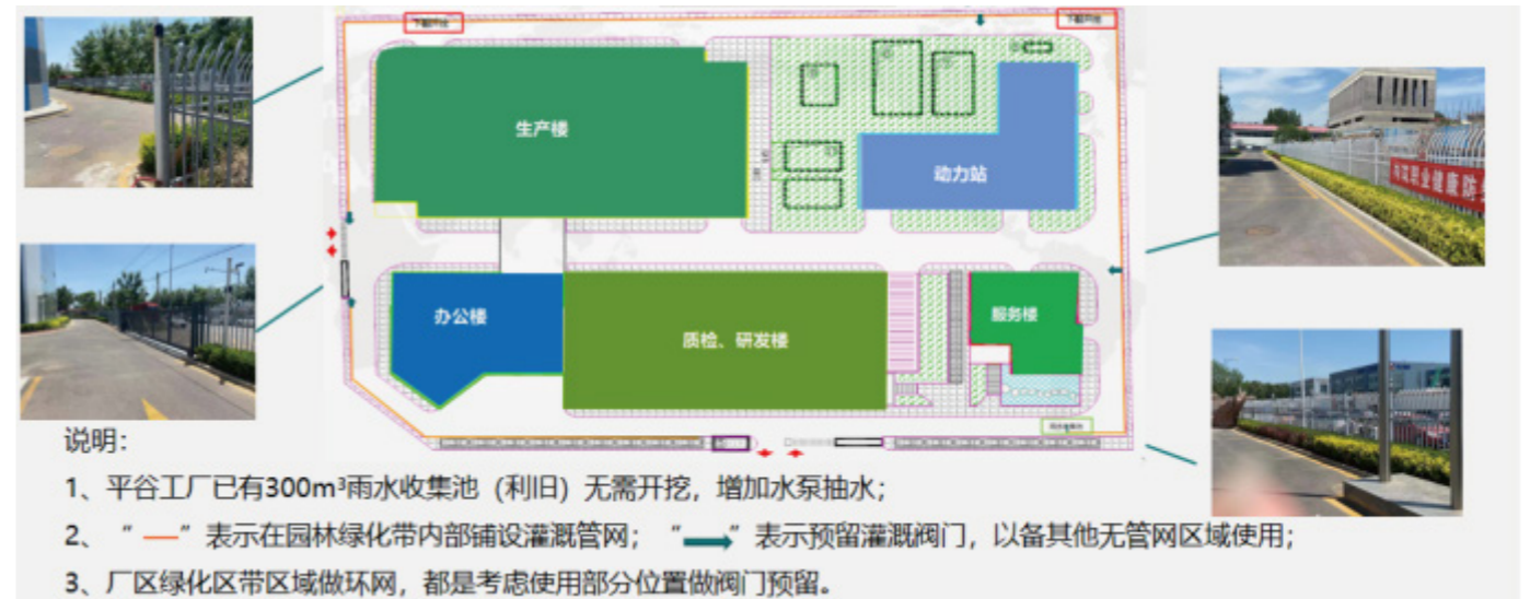
图注：雨水收集利用项目
