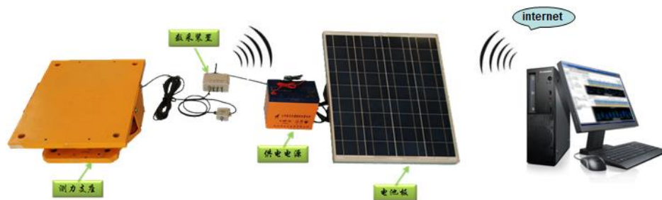
智能测力桥梁支座荷载监测系统示意图
