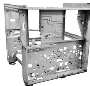
复印机框架
