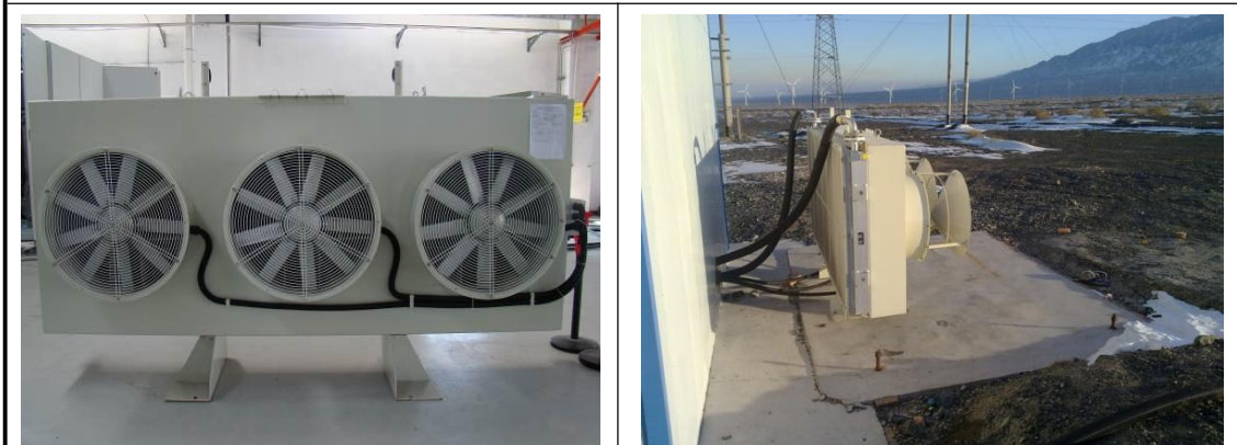
空冷器外观
