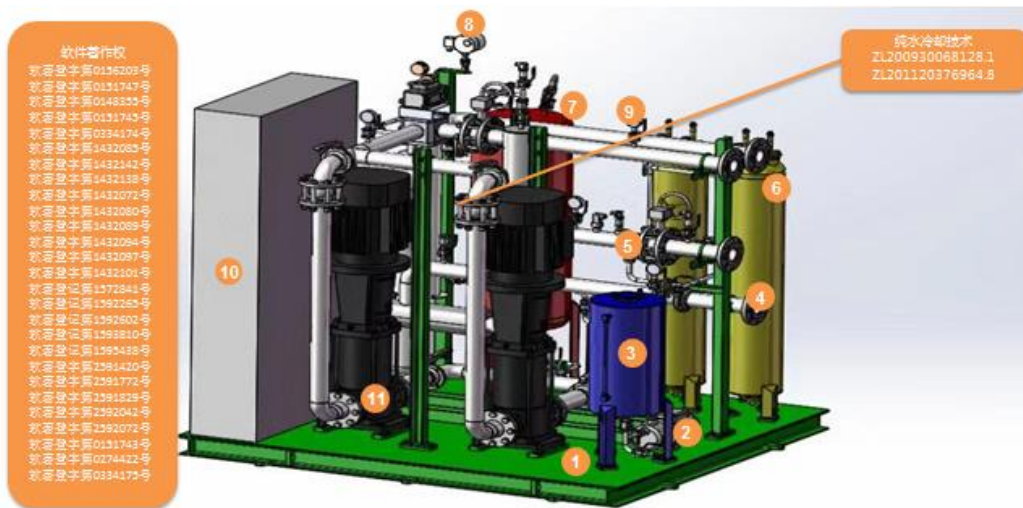
1.本体底座 2.补液泵 3.补水箱 4.主循环管道 5.副循环管道 6.离子罐 7.缓冲罐 8.氮气瓶稳压系统 9.仪器仪表 10.电控系统 11.水泵
