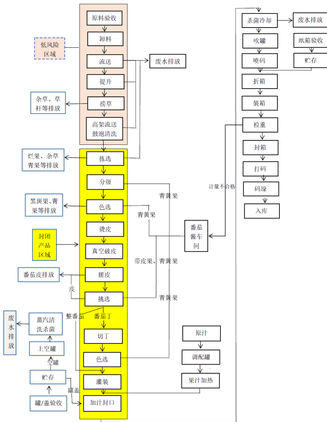
马口铁罐装去皮整番茄、番茄丁工艺流程图
