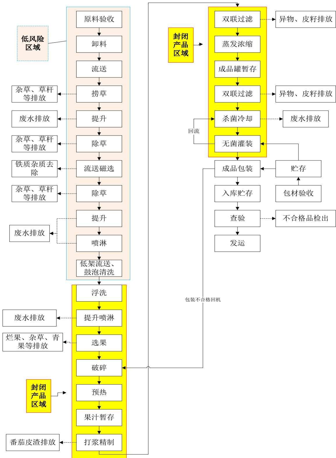
无菌袋装番茄酱工艺流程图
