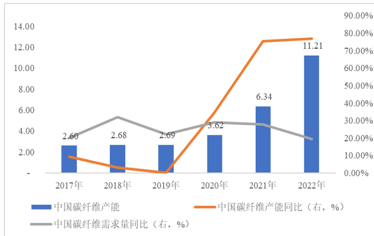
国内碳纤维产能及需求量增长情况（2017年-2022年）
