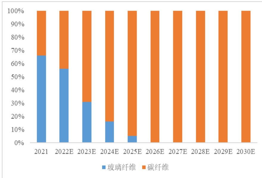
陆风：玻纤、碳纤维叶片主梁占比预测
