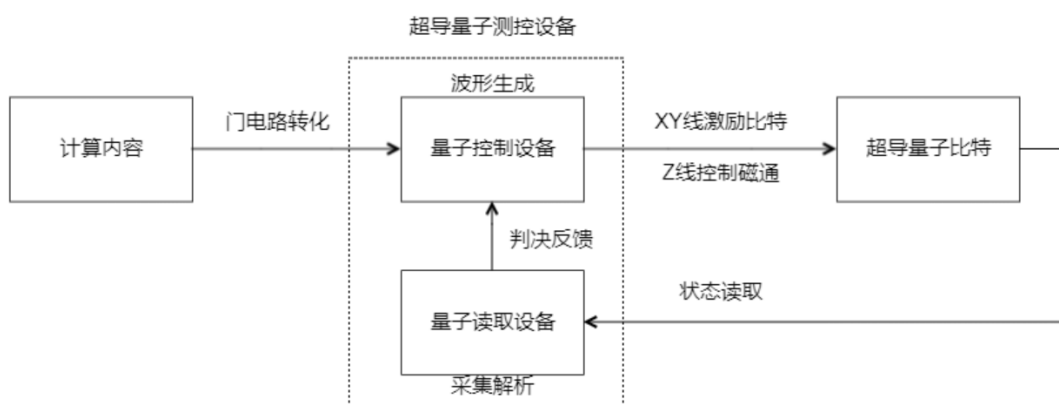
超导量子计算测控过程示意图
