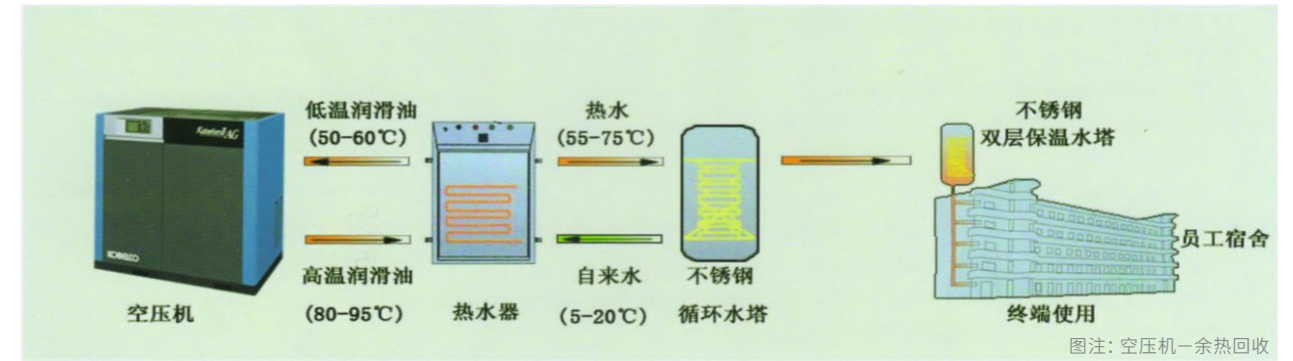
图注：空压机一余热回收
