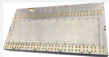
分布式相控节点 L 波段小型化多功能系统实物图
