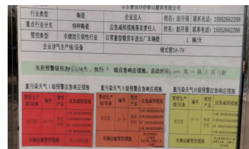
▲ 2023年重污染天气应急响应措施和机制
