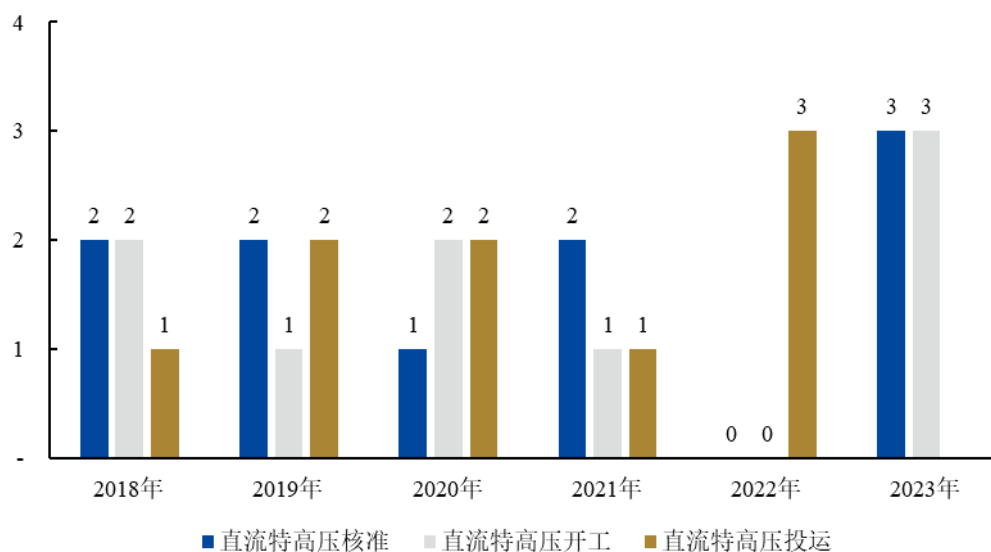
图表：我国特高压直流项目历年核准、开工、投运数量统计（单位：条）
