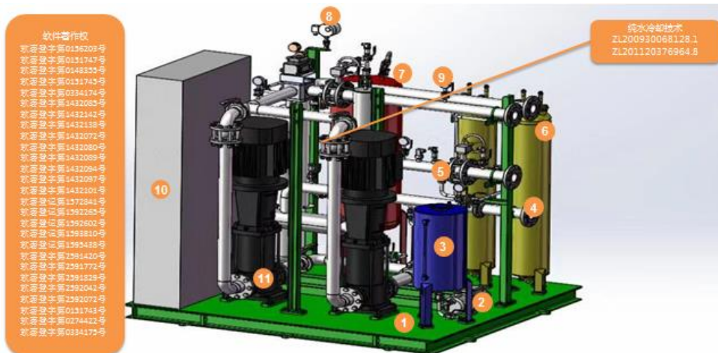
1.本体底座 2.补液泵 3.补水罐 4.主循环管道 5.副循环管道 6.离子罐 7.缓冲罐 8.氮气瓶稳压系统 9.仪器仪表 10. 电控系统 11.水泵
