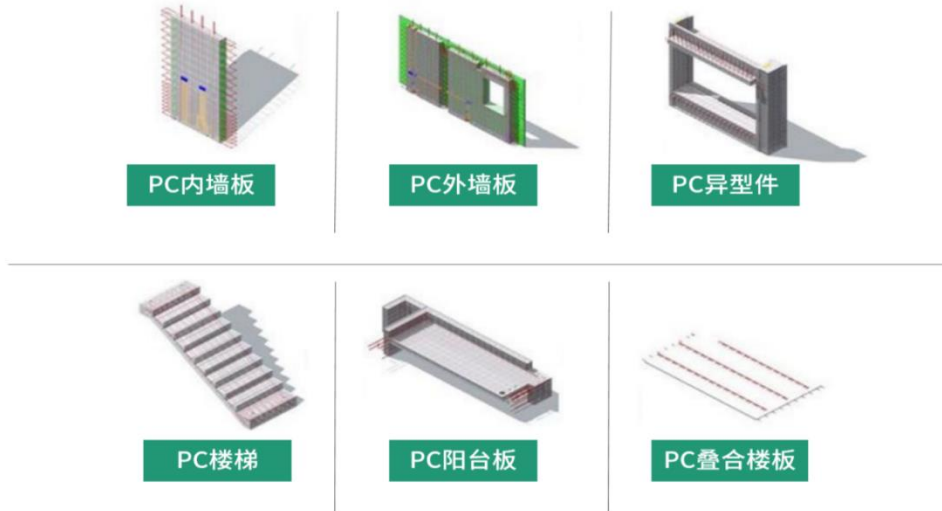
(图 2: PC 构件产品图)
